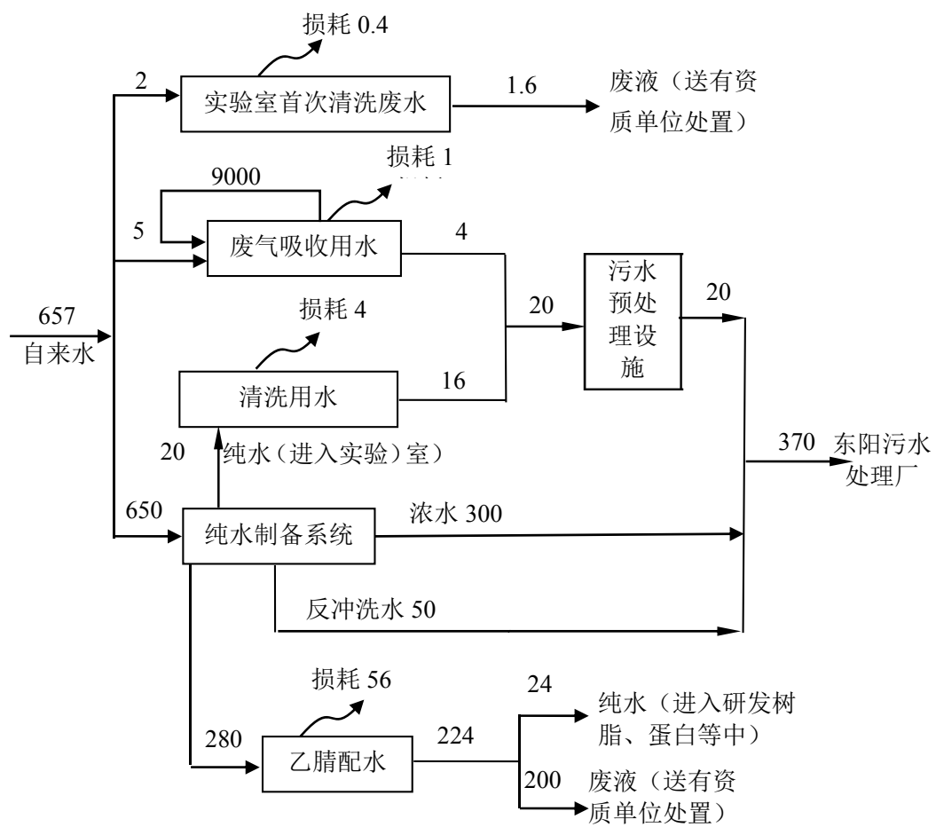
图 2-1 (a) 扩建项目用排水平衡图 (单位 t/a)
