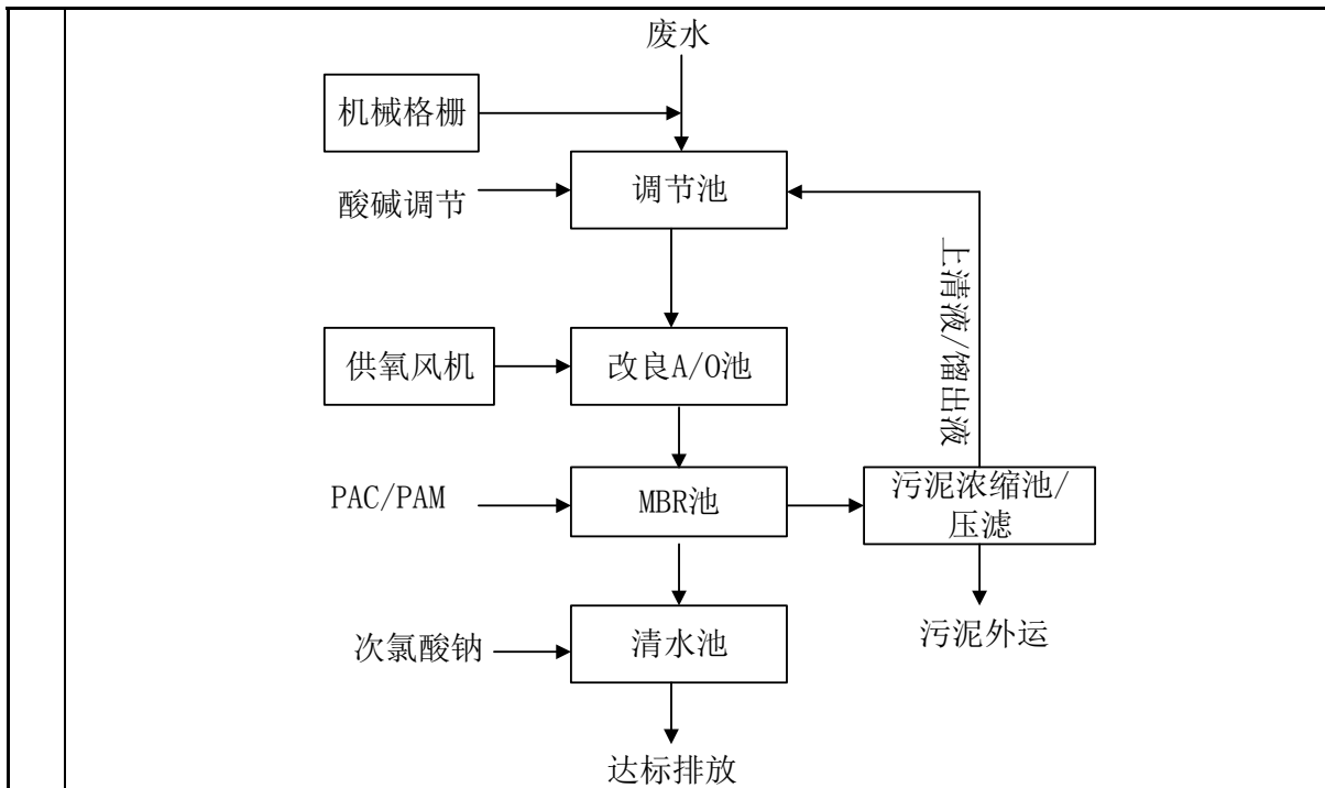
图 4-1 污水处理站工艺流程图
